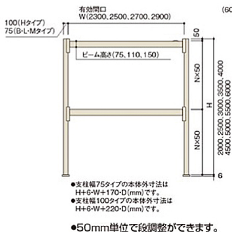
正面図
